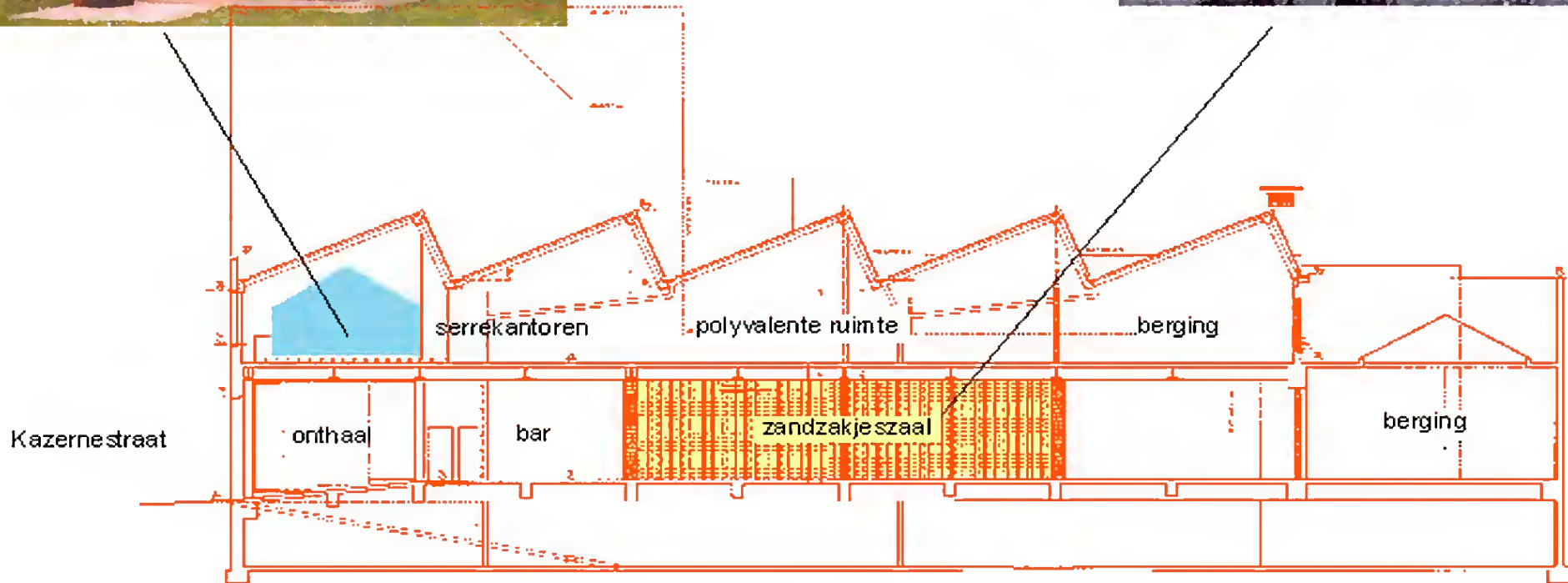
langse doorsnede
